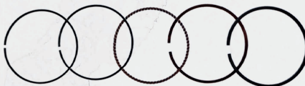
JOGO DE ANEIS GX100 | GXR120 | 5,5HP | 9HP | 13HP
